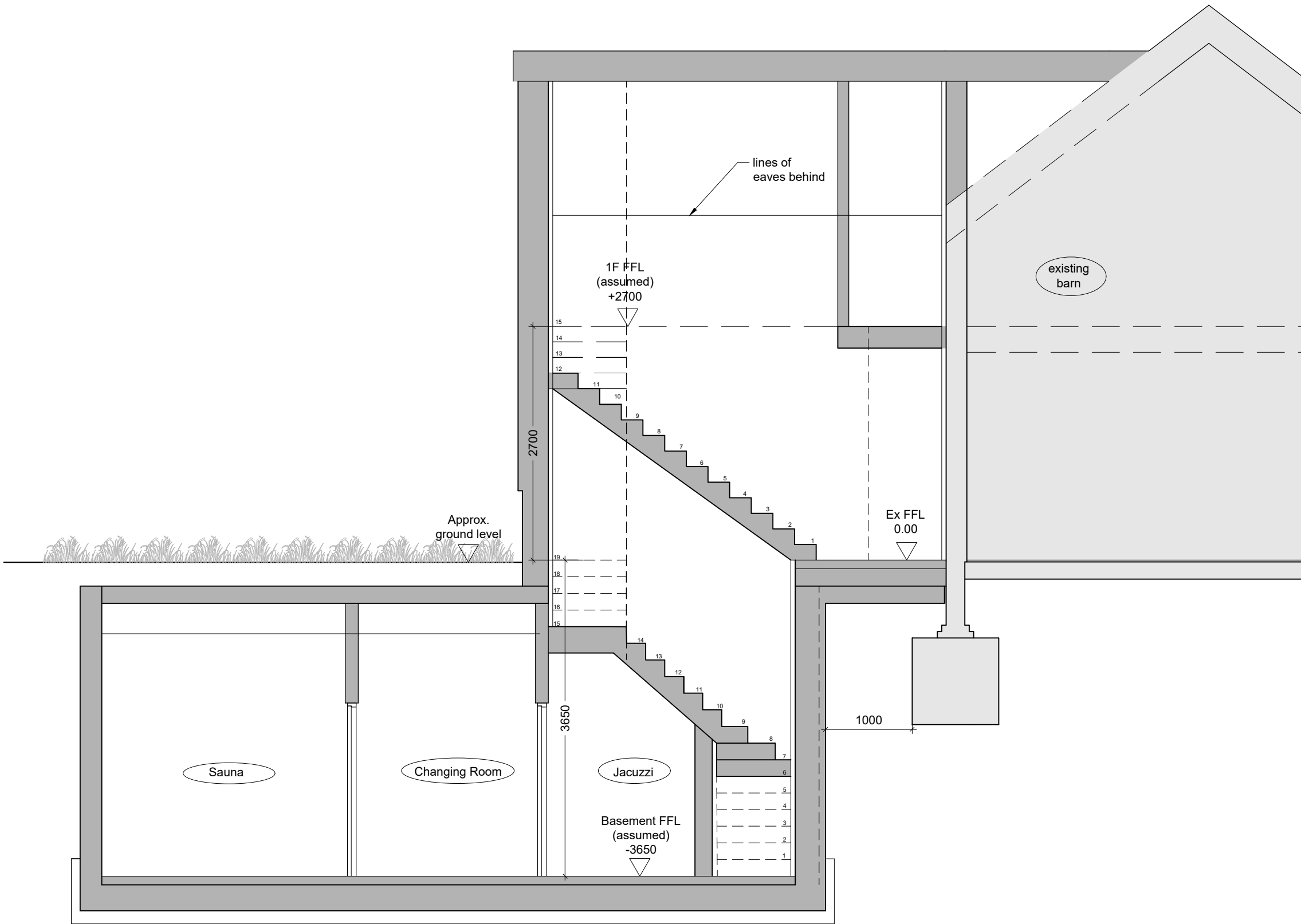
section a:a 1:50 @A3
